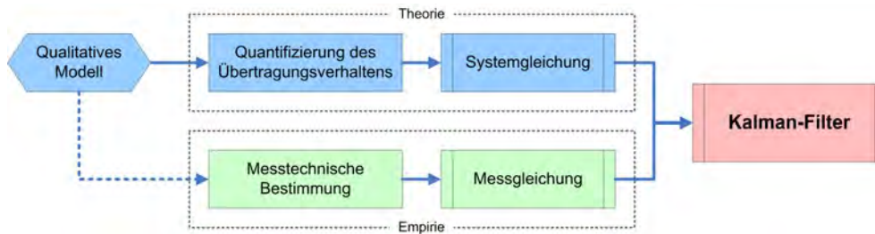
Abbildung 3.9: Zusammenführung von Mess- und Systemgleichung im Kalman-Filter (WELSCH u. a., 2000)
