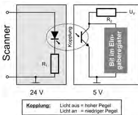
Abbildung 6.24: Pegelumsetzung
