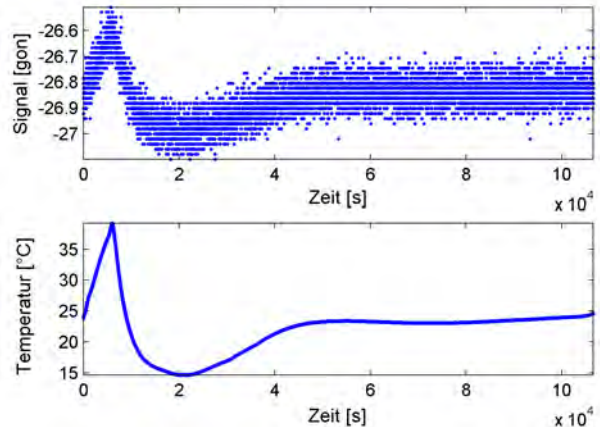
Abbildung 7.19: Signal- und Temperaturkurven bei -30° Neigung
