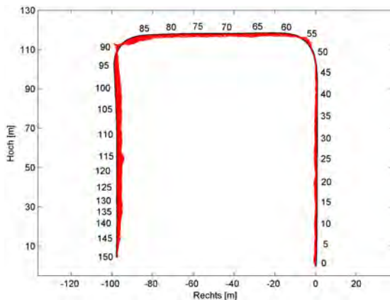
Abbildung 9.29: Abgefahrene Trajektorie mit Antennenposition
