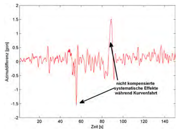
Abbildung 9.30: Azimutdifferenzen IMU-Filter
