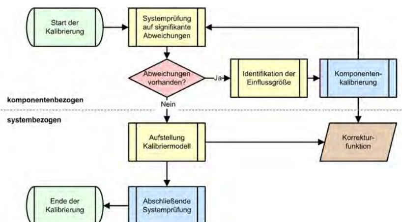
Abbildung 7.4: Kombination von Komponenten- und Systemkalibrierung
