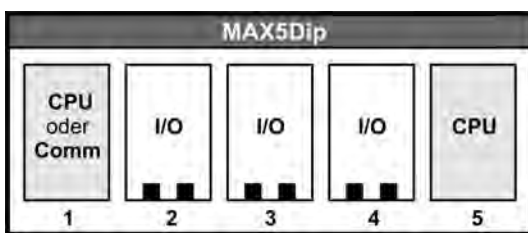
Abbildung 6.20: Steckplatzbelegung auf der MAX5dip
