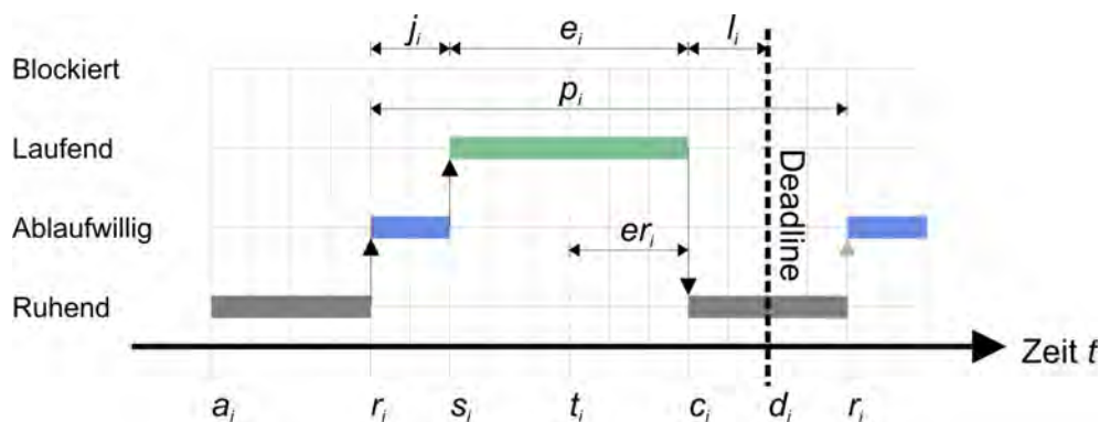
Abbildung 5.6: Zeitparameter einer Task
