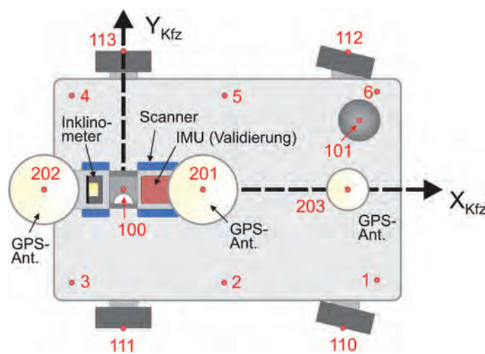
Abbildung 7.20: Fahrzeugkoordinatensystem
