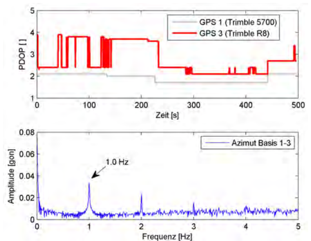
Abbildung 9.34: PDOP und Frequenzspektrum der Basis 1-3
