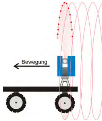
Abbildung 1.3: Helixförmige Objekterfassung
