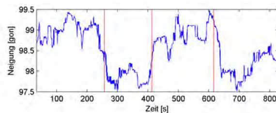
Abbildung 9.10: Neigungswerte der Teststrecke
