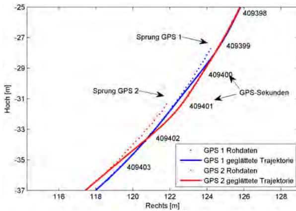
Abbildung 9.11: Versatz in den GPS-Beobachtungen
