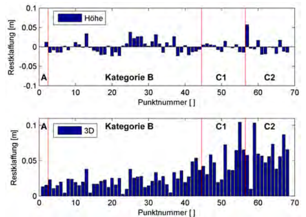
Abbildung 9.46: Restklaffungen der Höhe und Raumstrecke
