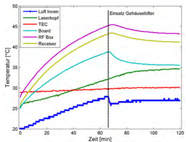
Abbildung 7.13: Temperaturverlauf Scanner
