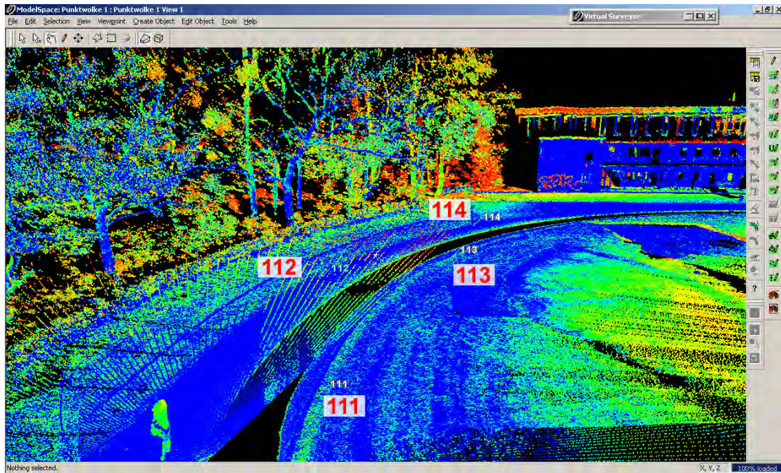
Abbildung 9.48: Punktübersicht mit abgeschatteten Zielmarken
