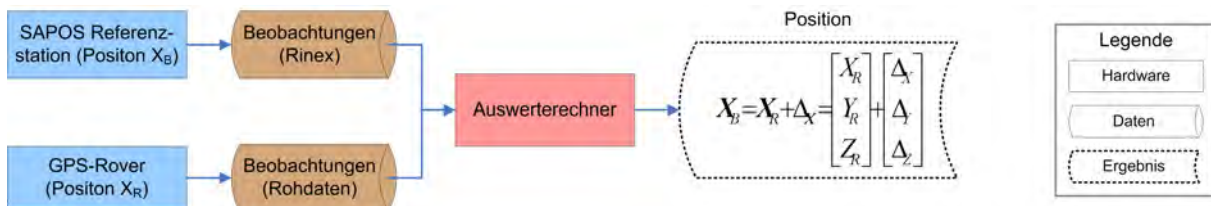
Abbildung 3.10: Prinzip der relativen GPS Bestimmung
