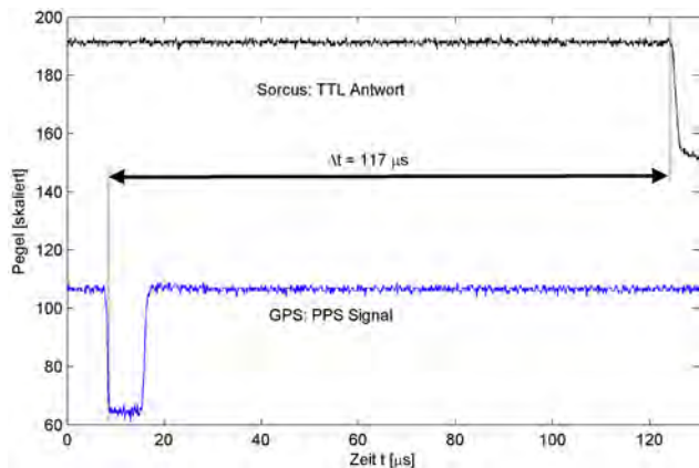
Abbildung 7.26: Latenzzeit bei hoher Systemlast
