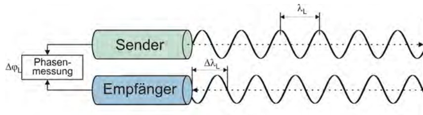
Abbildung 4.2: Phasenvergleichsverfahren
