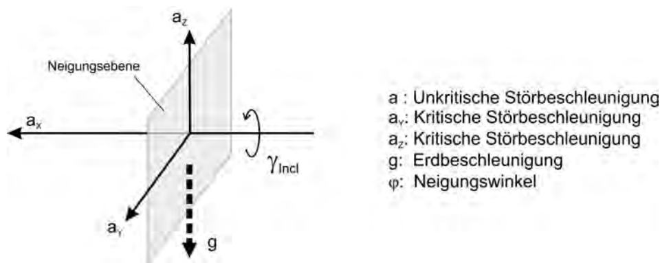
Abbildung 6.14: Einfluss von Störbeschleunigungen
