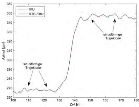
Abbildung 9.25: Azimute des Messwagens in der Übersicht
