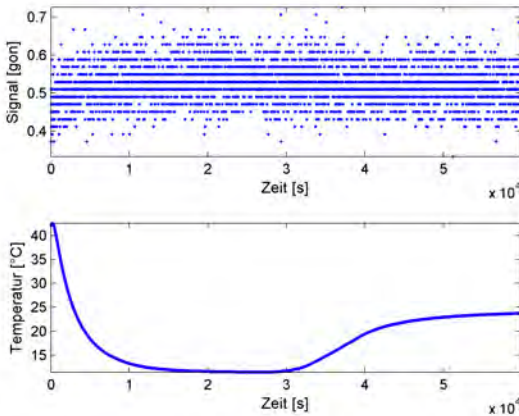
Abbildung 7.18: Signal- und Temperaturkurven bei 0° Neigung
