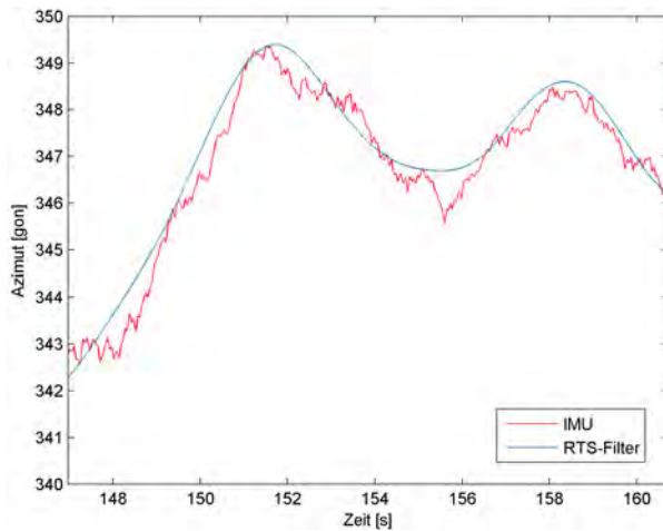
Abbildung 9.27: Azimute aus IMU und RTS-Filterung im Detail
