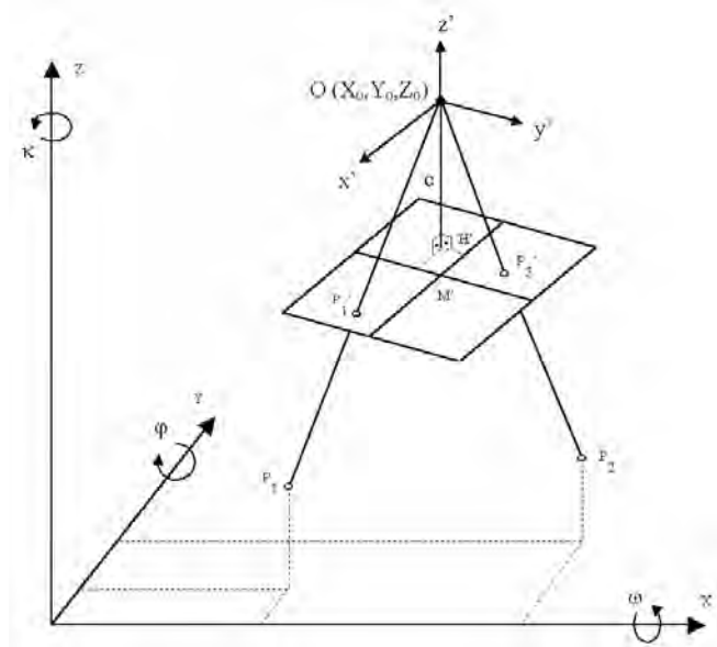
Abbildung 4.1: Geometrisches Modell der Zentralperspektive
