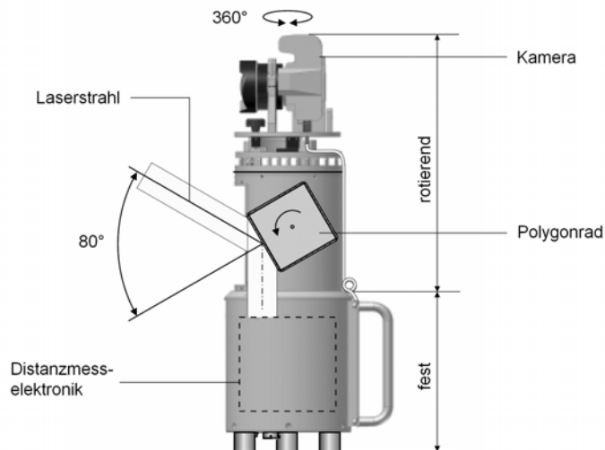
Abbildung 3.28: Aufbau des Laserscanners Riegl LMS-Z420i [Riegl, 2007]
