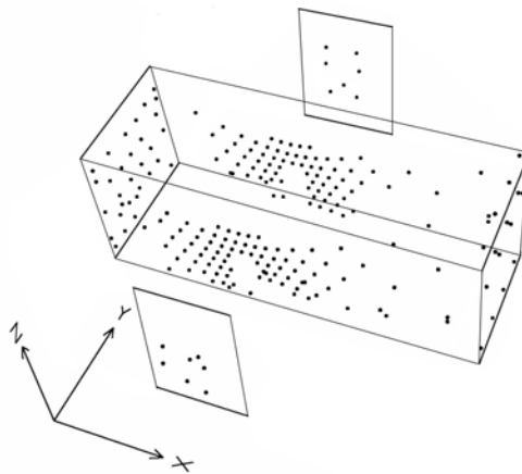
Abbildung 5.1: Kalibrierungsraum für Panoramakameras
