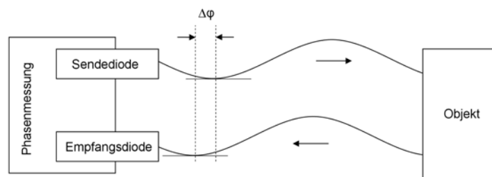
Abbildung 3.25: Prinzip des Phasenvergleichsverfahrens
