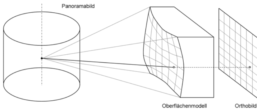
Abbildung 3.6: Prinzip der Orthobilderstellung aus einem 360°-Panorama
