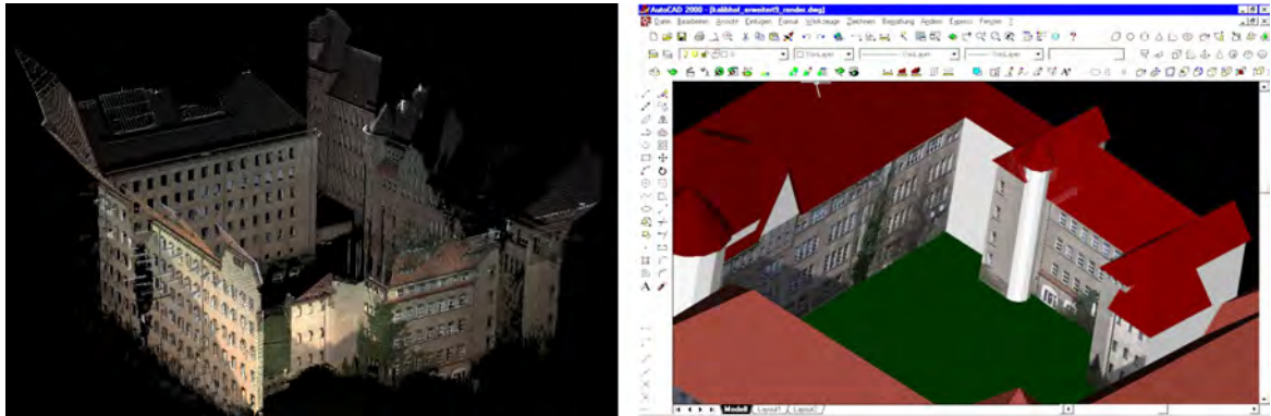
Abbildung A.17: Kolorierung einer Laserscanner-Punktwolke eines Innenhofes an der TU Dresden mit 360°-Panoramabildinformationen (links) und Generierung eines texturierten 3D-Modells mit AutoCAD (rechts) (vgl. Kapitel 5.1.3.3.)
