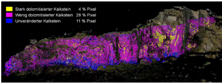
Abbildung A.19: Ergebnis für die geologische Interpretation: Punktwolke eingefärbt mit Klassifikationsergebnis der Hyperspektral-Panoramadaten, dargestellt über einem texturierten Oberflächenmodell (vgl. Kapitel 8.1.6.6) [Kurz et. al., 2008]
