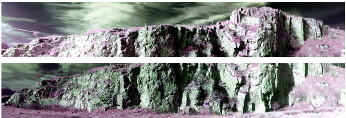
Abbildung A.18: Zwei Falschfarbenbilder (Rot: 1,720 \mu\text{m} , Grün: 2,009 \mu\text{m} , Blau: 1,563 \mu\text{m} ), erzeugt aus den Daten der hyperspektralen Panoramakamera HySpex SWIR-320m (vgl. Kapitel 8.1.6.2), aufgenommen von zwei vertikal übereinander angeordneten Standpunkten im 'Manystones' Steinbruch, Peak District (Großbritannien) (vgl. Kapitel 8.1.6.3) [Kurz et. al., 2008]
