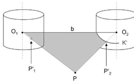
Abbildung 3.13: Panorama-Kernliniengeometrie
