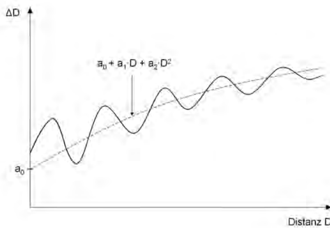
Abbildung 4.21: Schematische Darstellung möglicher Modellabweichungen der Distanzmessung terrestrischer Laserscanner
