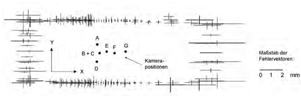
Abbildung 5.4: Grundriss des Kalibrierraumes: Kamerapositionen und Objektpunktgenauigkeiten
