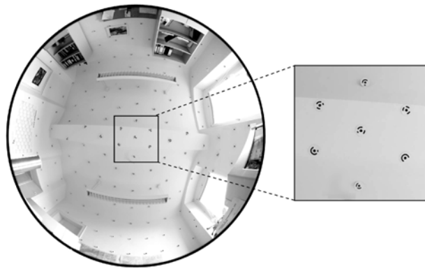
Abbildung 5.9: Kalibrierraum für Fisheye-Objektive [Schwalbe, 2005]
