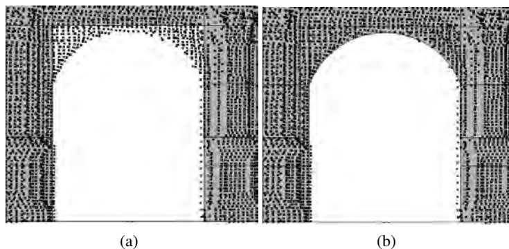
Abbildung 4.9: Überprüfung einer Rechtecksform: Zellerlegung und Fassadenpunkte (a), generierte Bogenform-Hypothese (b).
