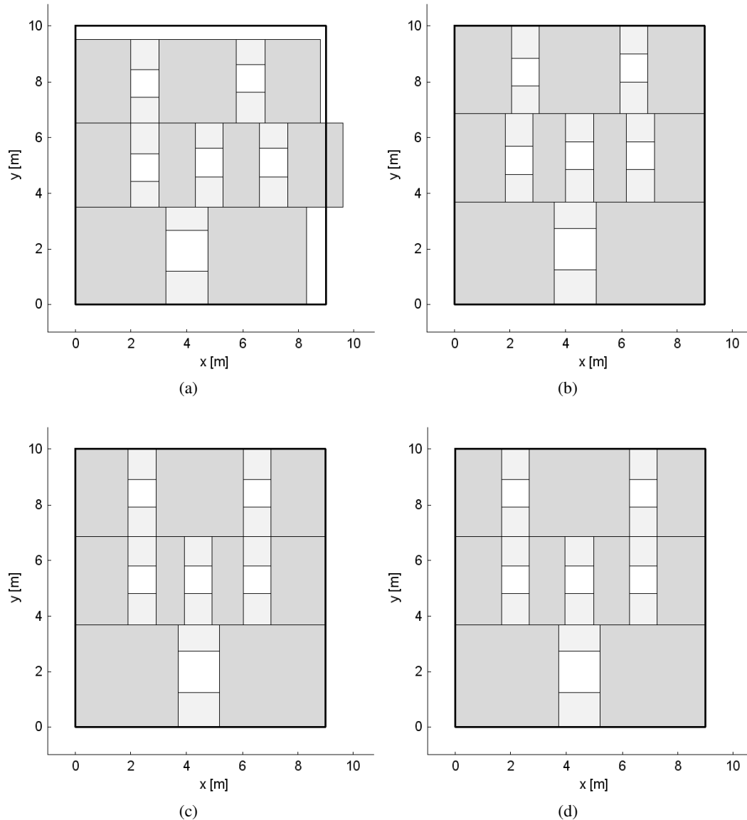
Abbildung 6.3: Geometrische Einpassung einer Kachelanordnung: Kachelanordnung vor der Ausgleiche (a), Ergebnis der Ausgleiche ohne Restriktionen (b), mit Gleichungsrestriktionen (c), mit Gleichungs- und Ungleichungsrestriktionen (d).
