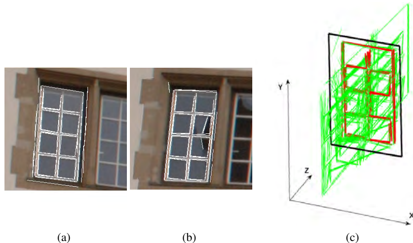
Abbildung 4.13: Datensatz „Alte Kanzlei, Stuttgart“: für ein bestimmtes Fenster selektierte 2D-Kanten im linken und rechten Foto (a) und (b) sowie die daraus abgeleiteten 3D-Kanten (c).
