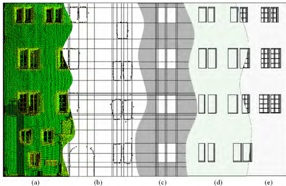
Abbildung 4.1: Unterschiedliche Stadien der datengetriebenen Fassadenrekonstruktion am Beispiel der Alten Kanzlei: LiDAR-Punktwolke (a), detektierte Kantenpunkte und -linien (b), klassifizierte Wandzellen (grau) und Fensterzellen (weiß) (c), 3D-Fassadenmodell (d), verfeinertes 3D-Fassadenmodell (e).
