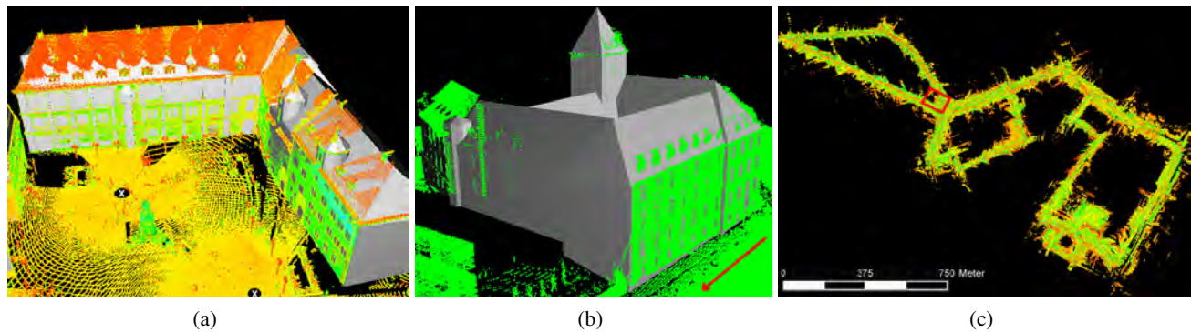
Abbildung 7.1: Typische Aufnahmekonfigurationen für statisches Laserscanning am Beispiel des Schillerplatzes (a) sowie für mobiles Laserscanning am Beispiel des Linden-Museums (b) (Fahrtrichtung durch Pfeil markiert); Übersicht über die mit dem StreetMapper in Stuttgart erfasste Punktwolke (c) (Bereich des Linden-Museums durch Polygon markiert).
