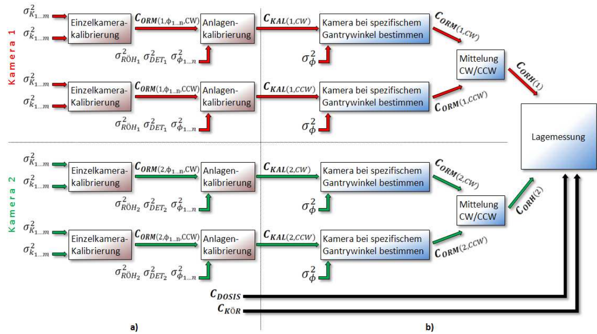
Abb. 5.3: Fehler der Kamerakalibrierung und ihrer Verwendung: a) Während der Kalibrierung gehen Unsicherheiten der m Kalibrierkugeln ein. Mit Ergebnissen für n Gantrywinkel werden Regressionsellipsen bestimmt (Anlagenkalibrierung); b) im Behandlungsbetrieb wird das Kameramodell für einen Gantrywinkel bestimmt. Rotationen im und gegen den Uhrzeigersinn werden gemittelt.
