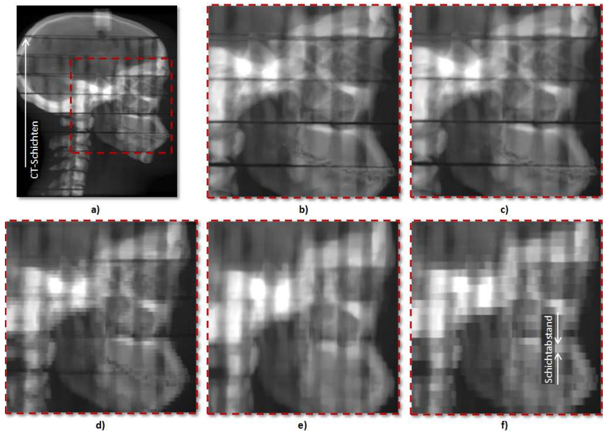
Abb. 7.13: DRRs unterschiedlicher Qualität für DS-6 (Anlage GTR-1): a) DRR für CT-Daten mit 0.625 mm Schichten, 1024^2 Bildraaster, trilineare Interpolation und b) vergrößerter Ausschnitt. Weitere Ausschnitte für c) 0.625 mm Schichten, 512^2 Raster, trilineare, d) 2.5 mm Schichten, 512^2 Raster, NN-, e) 5 mm Schichten, 512^2 Raster, trilineare und f) 5 mm, 512^2 Raster, NN-Interpolation.
