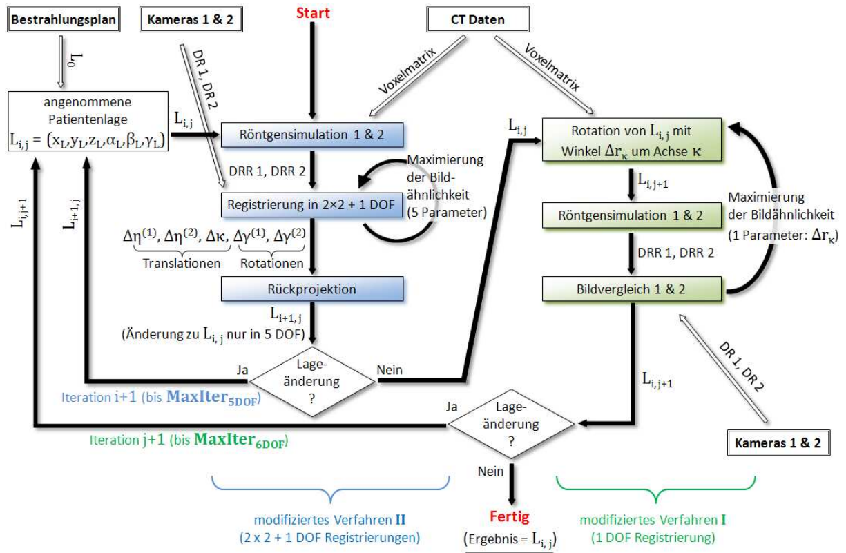
Abb. 4.10: Verfahren III zur Lagemessung: Das Verfahren besteht aus dem modifizierten Verfahren II , mit 2D-Registrierung und Rückwärtsprojektion, das in i Iterationen (links) und einem modifizierten Verfahren I , basierend auf Vorwärtsprojektion, das in j Iterationen durchlaufen wird (rechts).
