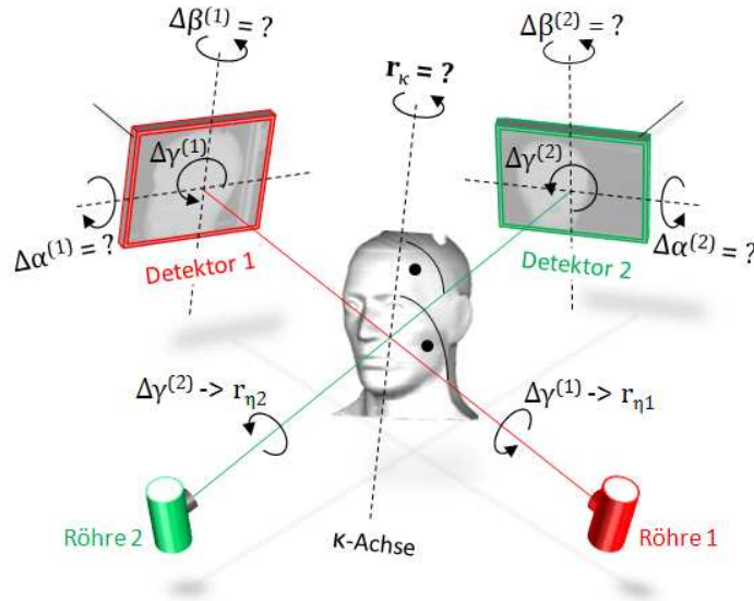
Abb. 4.8: Aus 2D-Registrierungen ermittelbare Rotationen: Rotationen \Delta\gamma^{(1)} und \Delta\gamma^{(2)} in den Ebenen erlauben lediglich die Bestimmung zweier Komponenten r_{\eta_1} und r_{\eta_2} der räumlichen Orientierung.
