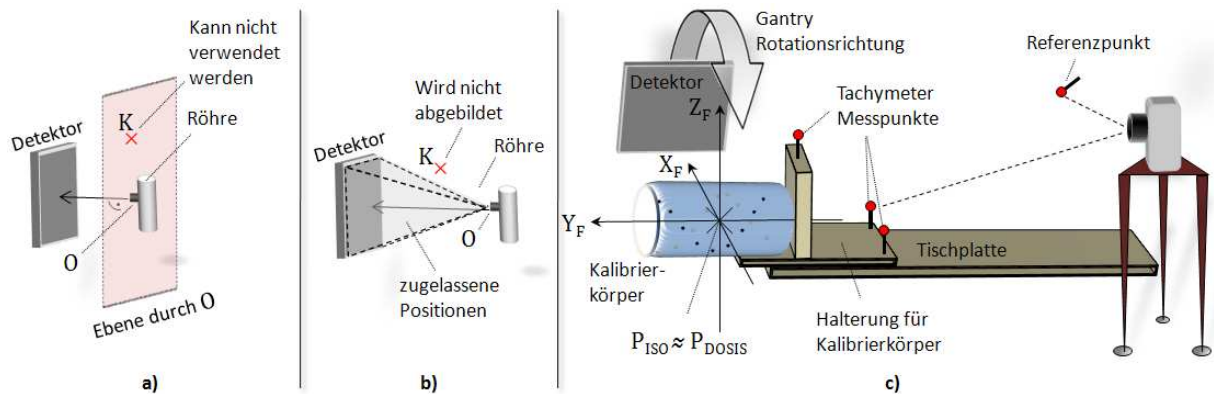
Abb. 3.5: Problematische Kugelpositionen und Ausrichtung eines Kalibrierkörpers: a) Bestimmte Positionen eignen sich rechnerisch oder b) physikalisch nicht zur Kalibrierung; c) ein Kalibrierkörper wird auf dem Patiententisch mittels Tachymeter ausgerichtet.
