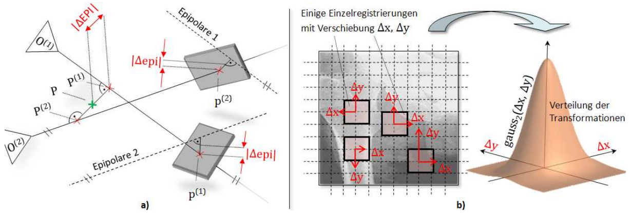
Abb. 5.6: Geometrie- und Registrierfehler: a) Verstoß gegen die Epipolargeometrie mit Fehler \Delta EPI ; b) DR-DRR Registrierung von mehreren Teilflächen zur Bestimmung von Translationen \Delta x , \Delta y (links) sowie Verteilung redundanter Registrierergebnisse (rechts).
