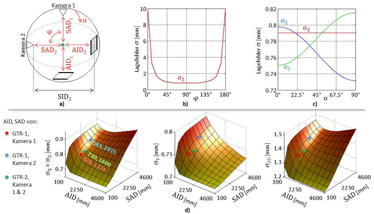
Abb. 7.25: Fehler bei geänderter Anlagengeometrie: a) Skizze verwendeter Geometrieparameter, b) \sigma_z -Fehler über \phi , c) Fehler über Verkippung der Anlage und d) Fehler über unterschiedliche Werte der Abstände AID und SAD für beide Kameras.
