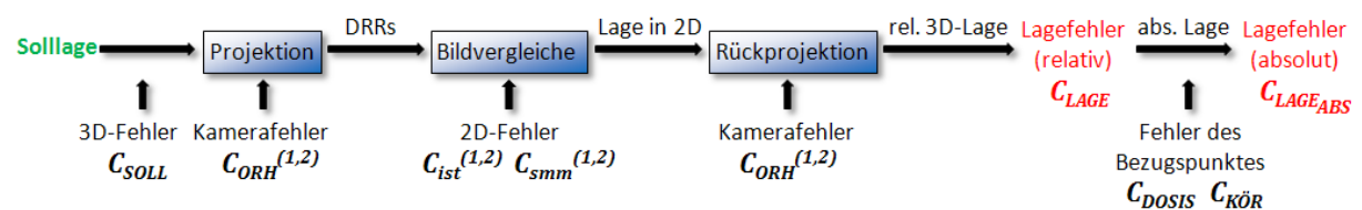
Abb. 5.4: Konzept zur Bestimmung des Lagefehlers: Die Solllage (mit C_{SOLL} ) wird mit fehlerbehafteten Kameramodellen ( C_{ORH} ) projiziert. In den Bildebenen kommen 2D-Fehler ( C_{ist} , C_{smm} ) hinzu. Bei der Rückprojektion werden wieder fehlerbehaftete Kameramodelle verwendet. Fehler des Bezugspunktes für die Lagemessung werden durch C_{DOSIS} und C_{KÖR} berücksichtigt.
