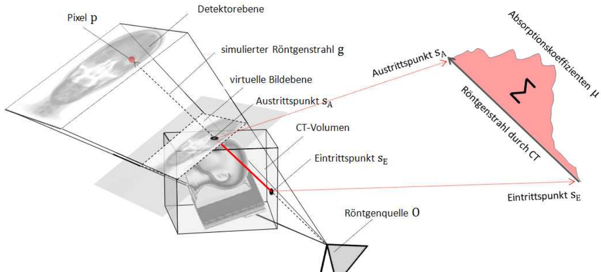
Abb. 4.12: Simulation von Röntgenbildern mittels Raytracing: Für alle Bildpunkte der virtuellen Bildebene werden Strahlen von der angenommenen Position der Röntgenquelle bestimmt. Bei der Strahlverfolgung werden die entsprechenden Absorptionskoeffizienten aufsummiert (rechts).
