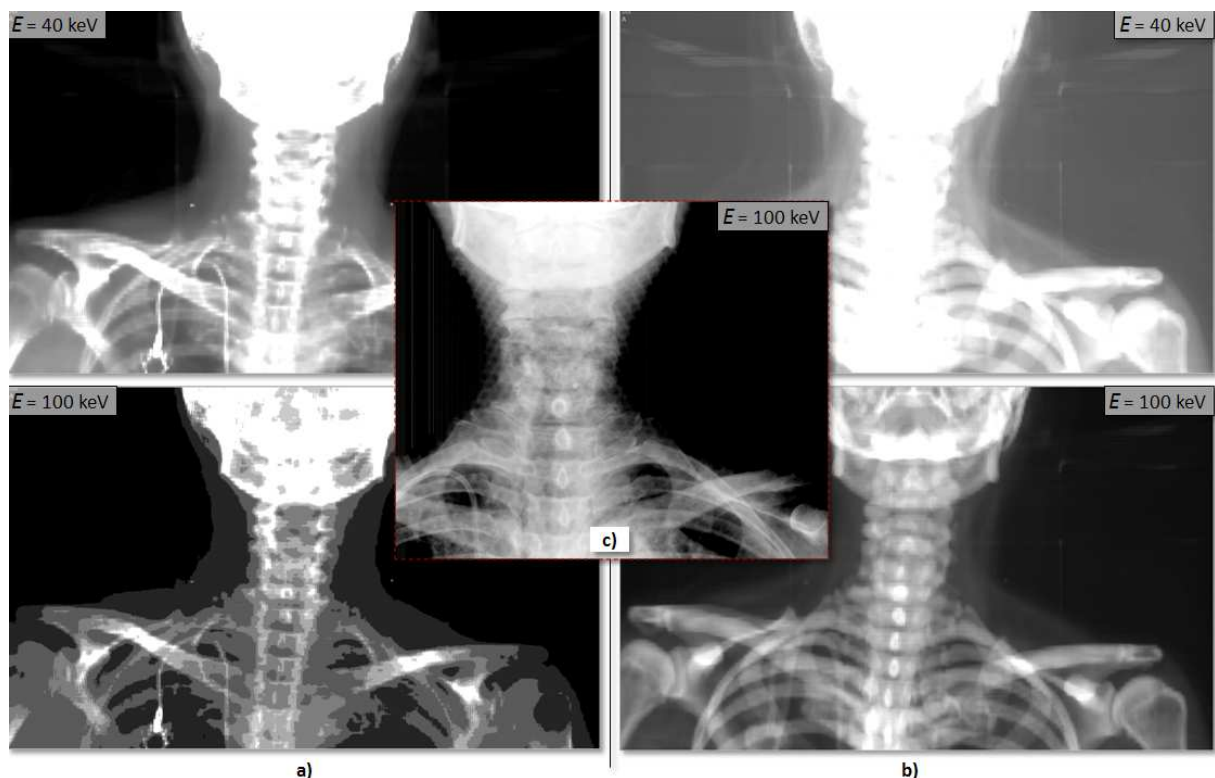
Abb. 7.15: Unterschiedliche Radiometriesimulation: Bilder von Thoraxpatient DS-5 für 40 keV bzw. 100 keV Maximalenergie. a) DRRs mit Absorptionen direkt aus CT-Zahlen, b) DRRs mit Materialgewichtung und c) 100 keV Röntgenbild (frontale Ansicht, überlagert von einem Fixiernetz auf dem Gesicht des Patienten).
