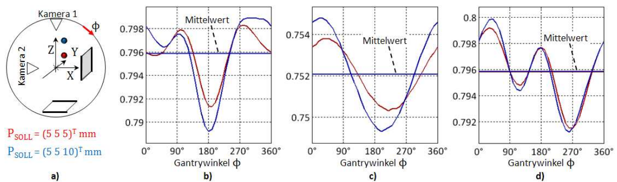
Abb. 7.23: Theoretischer Lagefehler bei verschiedenen Gantrywinkeln in GTR-1: a) Skizze der Geometrie, b) Standardabweichungen der Lage in X-, c) in Y- und d) in Z-Richtung für zwei verschiedene Sollagen (Kurven in rot und blau).
