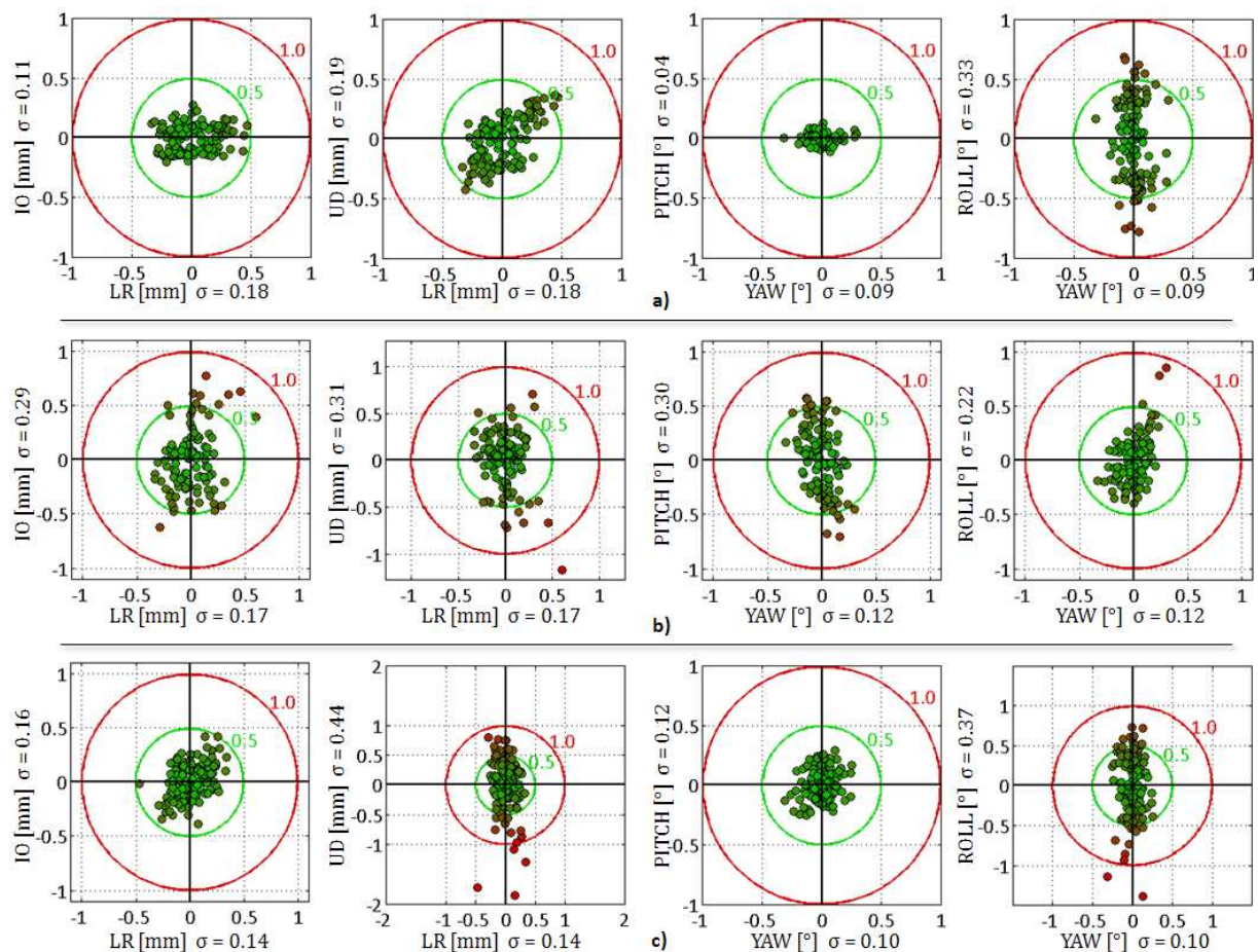
Abb. 7.19: Streudiagramme zur Präzision erfolgreicher Lagemessungen: Vergleich verschiedener Freiheitsgrade, a) für Kopfphantom DS-1, b) Prostatapatienten DS-2 und c) Kopfpatienten DS-3.
