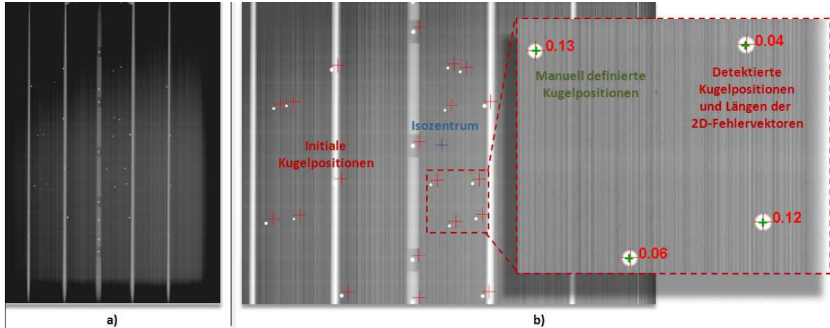
Abb. 7.2: Kugeldetektion im Kalibrierbild: a) Röntgenbild des Kalibrierkörpers mit konstruktionsbedingten Artefakten (vertikale Streifen), b) Ausschnitt mit genäherten Kugelprojektionen und (in der Vergrößerung, rechts) Fehler nach Kugeldetektion (grün: manuell definierte Kugelpositionen, rot: detektierte Kugelpositionen und Fehlerwerte in mm).
