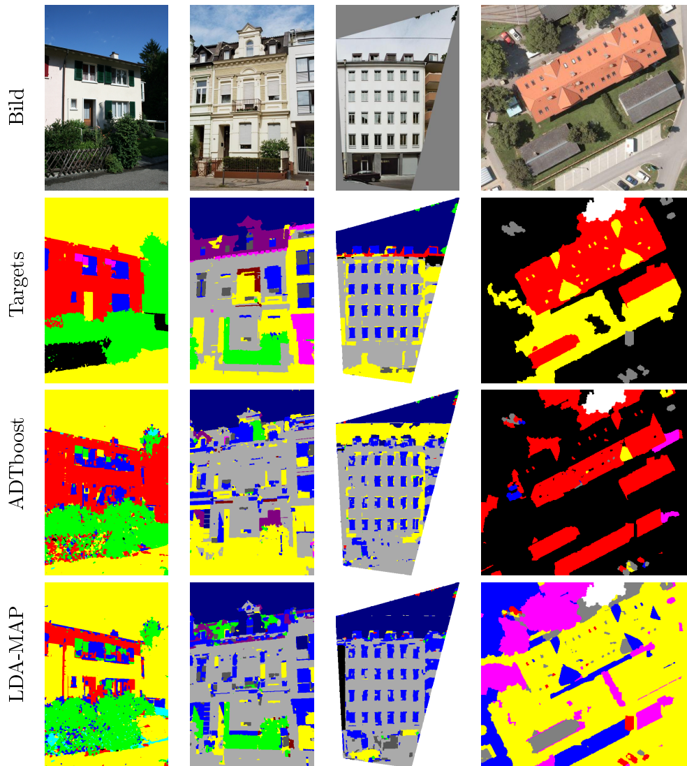
Abbildung 4.22.: Visueller Vergleich zwischen den Targets der Regionen und den Klassifikationsergebnissen für die Beispielbilder aus Abb. 2.14, die wir noch einmal in der obersten Zeile zeigen. Darunter visualisieren wir erneut die Targets der Regionen (wie in Abb. 3.9). Die beiden unteren Zeilen sind neu, darin präsentieren wir die Klassifikationsergebnisse mit ADTboost sowie mit der MAP-Klassifikation im LDA-Unterraum. Vertikal gesehen bedeuten gleiche Farben auch gleiche Klassen. Weiße Pixel bedeuten dabei, dass in diesem Bildbereich keine stabilen Regionen segmentiert und daher auch nicht klassifiziert wurden. Schwarz sind alle Pixel, die als stabile Region in nicht annotierten Bereichen segmentiert wurden, d. h. sie gehören zur Klasse background . In den terrestrischen Aufnahmen wird Vegetation grün, die Fenster blau, die Restklasse gelb dargestellt, in der linken Spalte bedeutet rot Gebäude, in der Mitte grau Fassade. In den Luftbildern haben wir die Dächer rot visualisiert.
