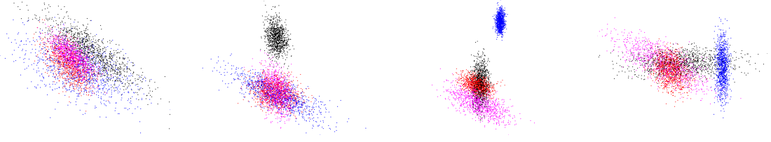
Abbildung 4.17.: Visualisierung des Datensatzes von Fukunaga (1972). V. l. n. r. zeigen wir jeweils zwei verschiedene Merkmale des 8D-Merkmalraums, u. z. die Merkmale f_1 und f_2 in im linken Plot, f_3 und f_4 rechts daneben etc.
