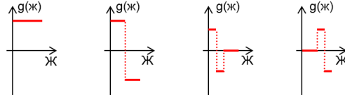
Abbildung 4.6.: Eindimensionale Haar-Funktionen.
