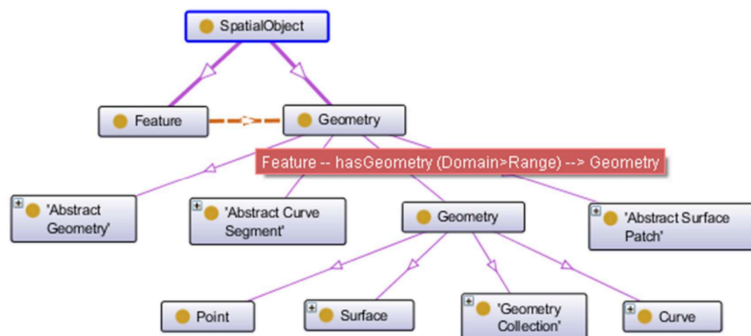
Abbildung 18: Darstellung des GeoSPARQL-Vokabulars und deren Beziehungen als Ontologie-Graph (Würriehausen, Karmacharya & Müller, 2014)
