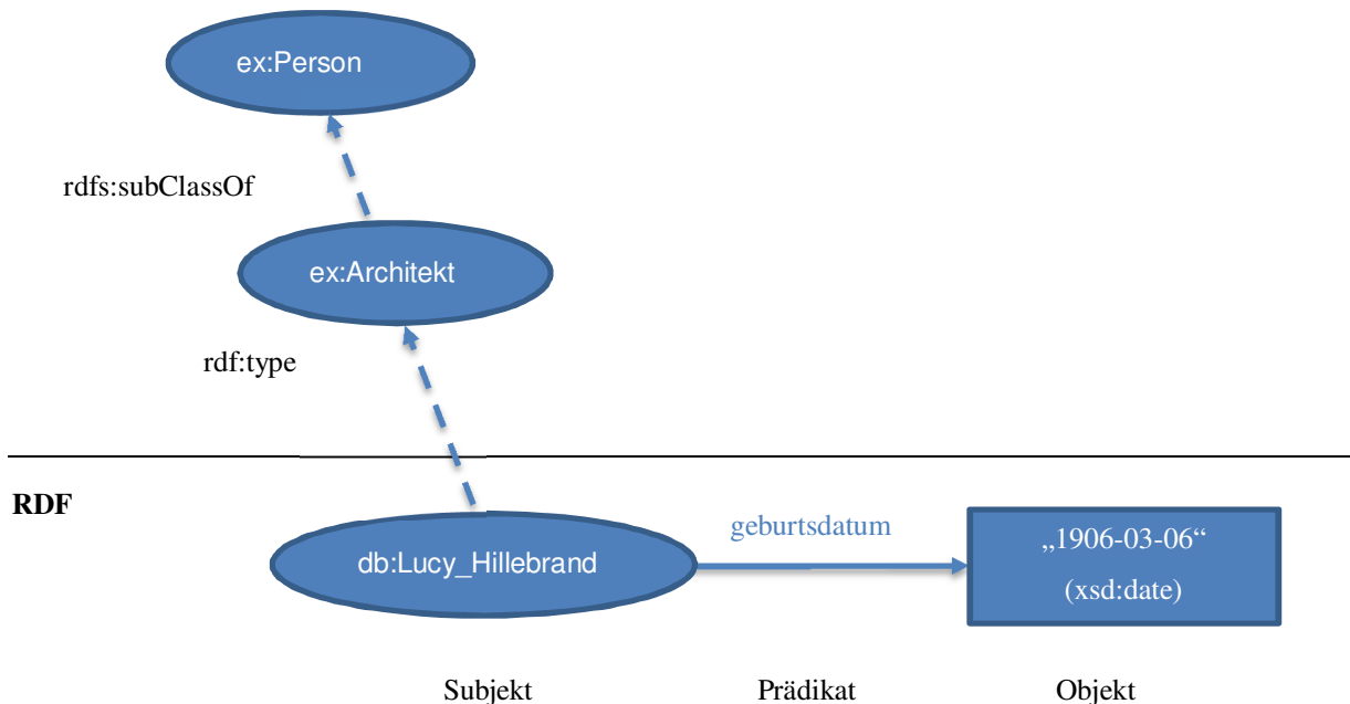
Abbildung 17: Abgrenzung RDFS von RDF-Triples, Lucy Hillebrand als Person
