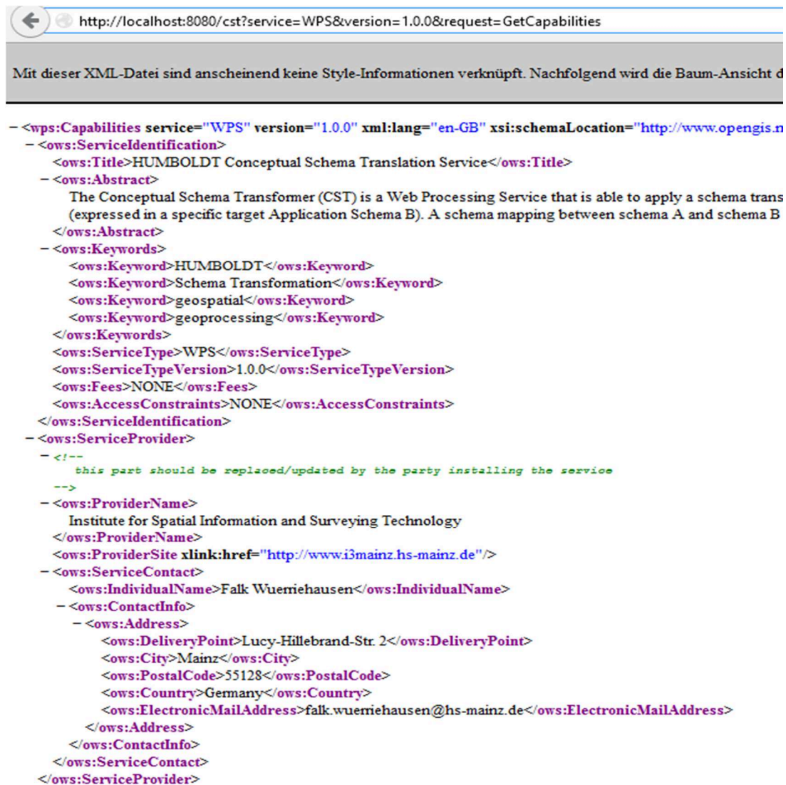
Abbildung 51: CST-WPS Service, eigene Implementierung
