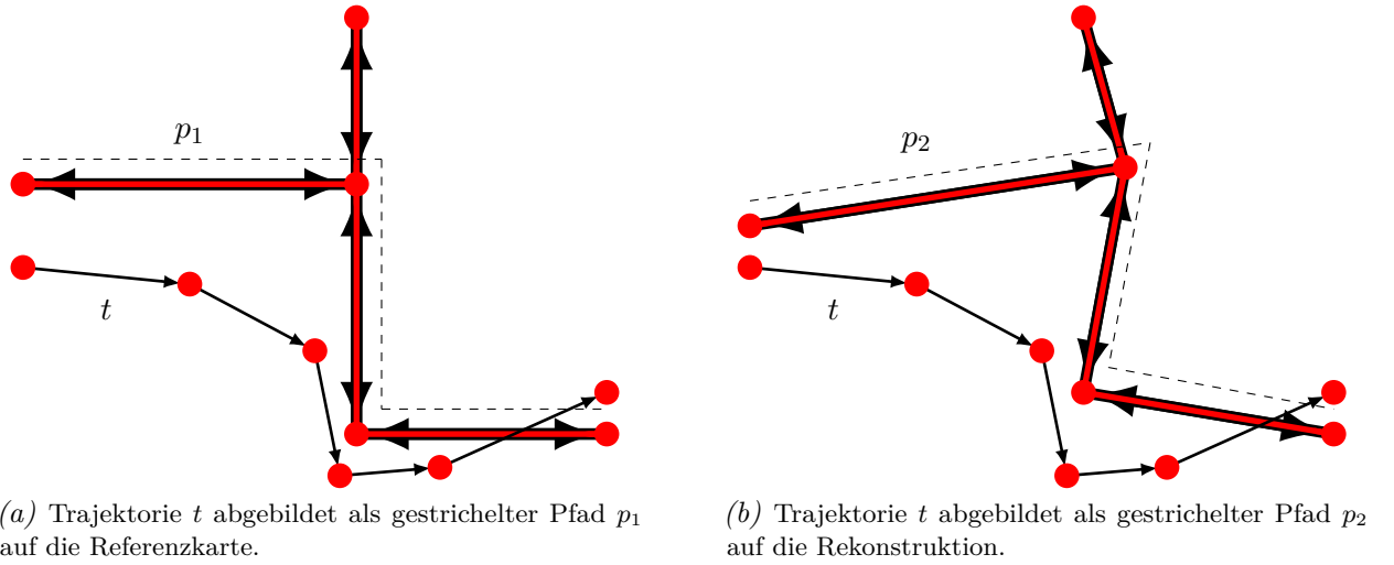
Abbildung 6.7.: Die Pfadlängen-Differenz.
