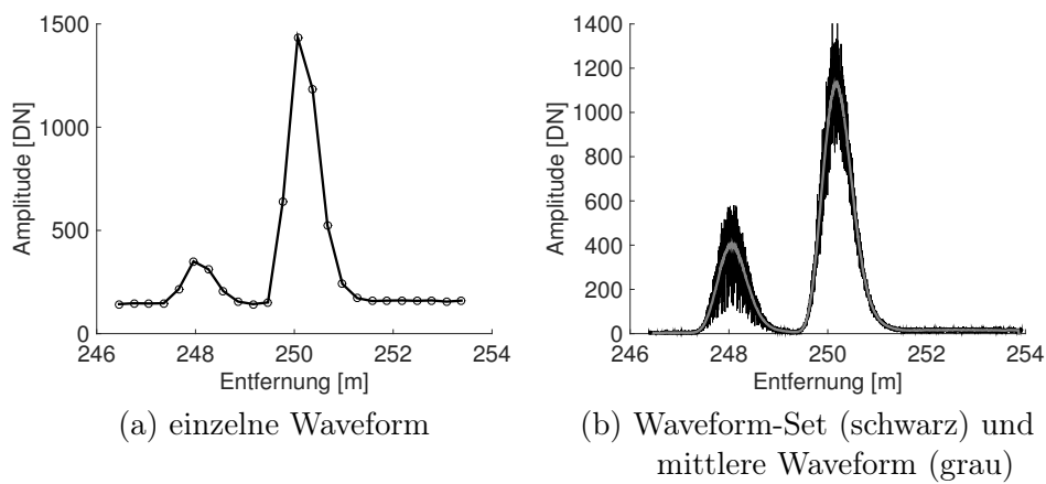
Abbildung 8.6: Extrahierte Waveforms für das Szenario Platte auf P3 und Gitter auf P1
