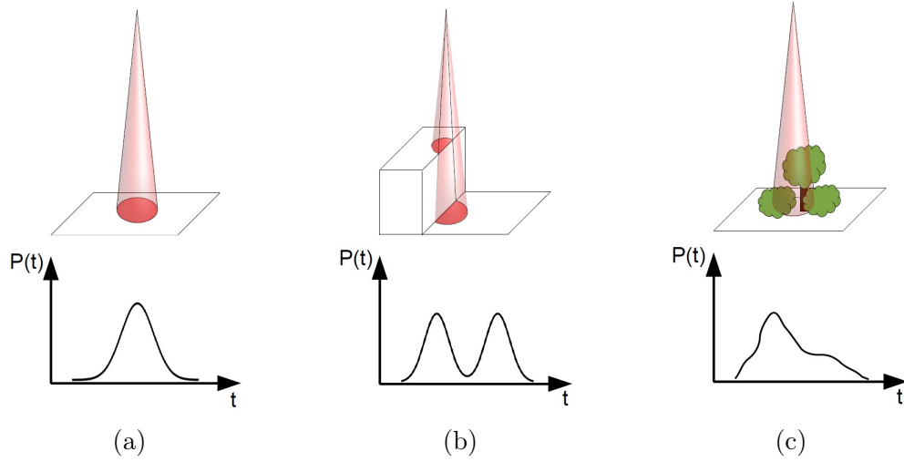
Abbildung 2.5: Unterschiedliche Ziele mit resultierender Signalforn. (a) ausgedehntes ebenes Ziel, (b) zwei ebene Teilziele, (c) Volumenstreuer Vegetation. (Abbildung in Anlehnung an Jutzi (2007))
