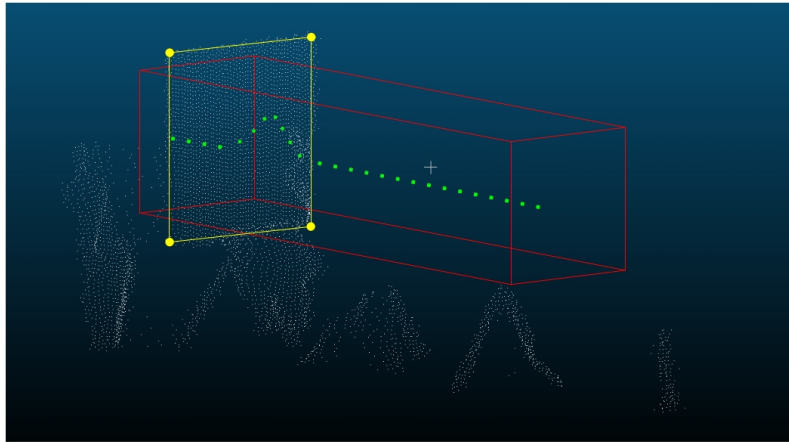
Abbildung 8.5: Definition des Volumens für die Extraktion der Waveforms des Baummodells, Punktwolke Platte (weiß), Eckpunkte Platte (gelb), Volumen (rot), Beispielwaveform mit Interaktion an der Platte (grün)
