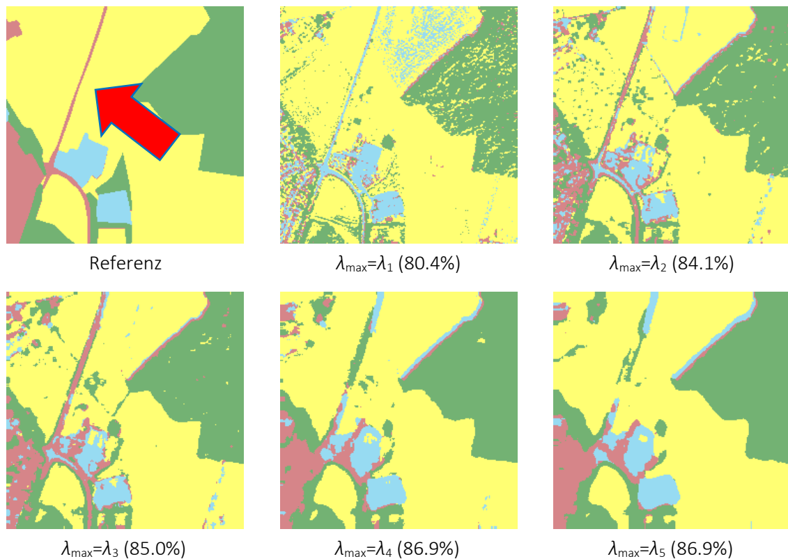
Abbildung 5-7: ML-Klassifikationsgenauigkeit von Ikonos-Daten in Abhängigkeit der verwendeten maximalen Skala \lambda_{\max} für die Merkmalsselektion – Region 2.
