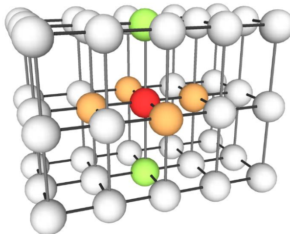
Abbildung 4-2: Graphstruktur für die Klassifikation mehrerer Bilder mit identischer geometrischer Auflösung. Roter Knoten: Betrachtetes Pixel; Orange Knoten: Pixel in räumlicher Nachbarschaft zum betrachteten Pixel; Grüne Knoten: Pixel in zeitlicher Nachbarschaft zum betrachteten Pixel.
