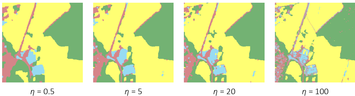
Abbildung 5-9: Klassifikationsergebnisse für IS_3 mit \lambda_{\max}=\lambda_1 für h_i^t(y^t) in Abhängigkeit von \eta . Bilddaten: Ikonos (240*240 Pixel), \beta = 0.7 .
