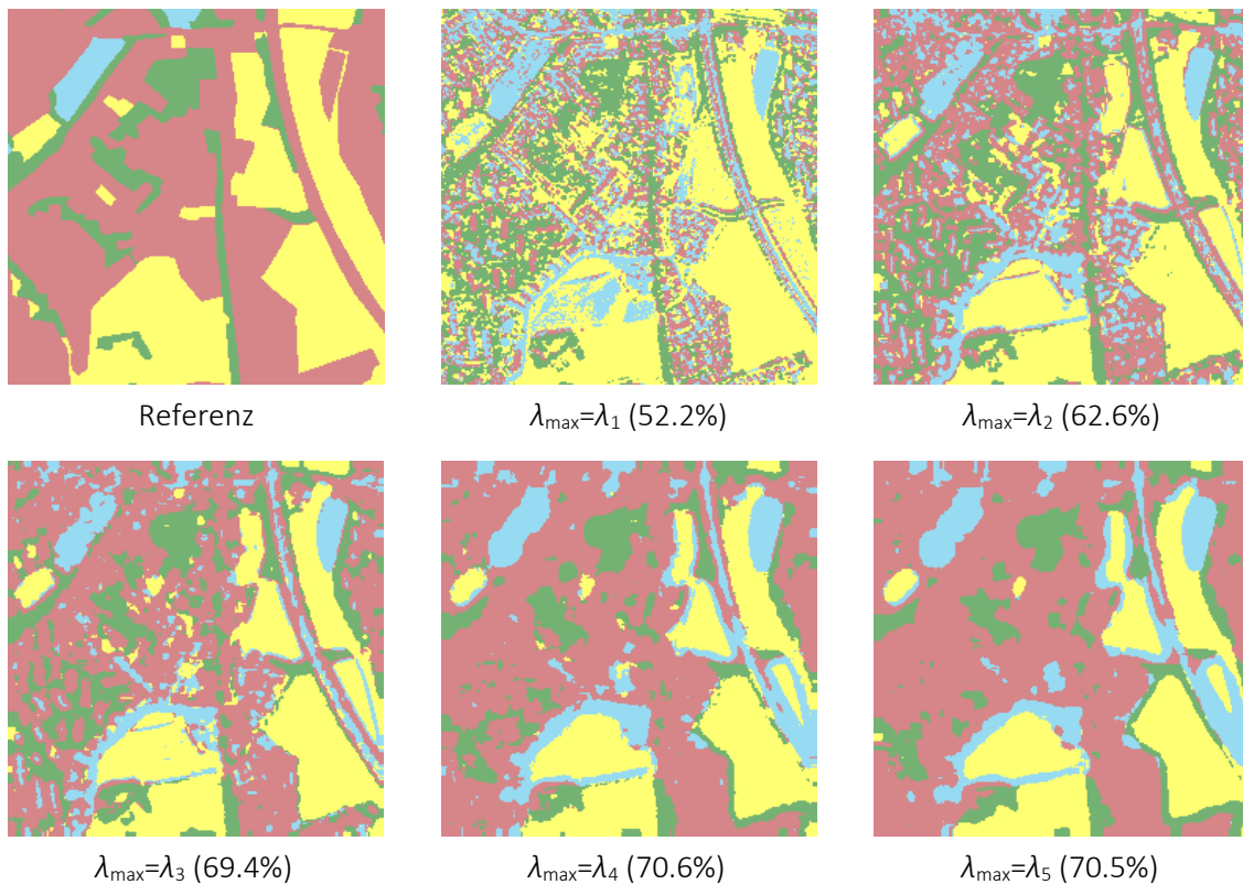
Abbildung 5-8: ML-Klassifikationsgenauigkeit von Ikonos-Daten in Abhängigkeit der verwendeten maximalen Skala \lambda_{\max} für die Merkmalsselektion – Region 3.
