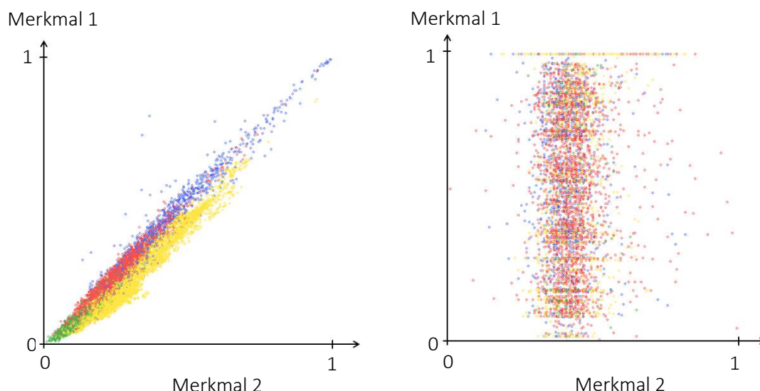
Abbildung 3-2: Scatter Plot für 4 Klassen von zwei hoch korrelierten Merkmalen (links) und zwei schlecht trennenden Merkmalen (rechts). Die Merkmale wurden auf den Wertebereich [0;1] normalisiert.
