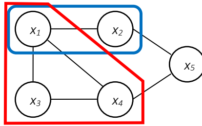
Abbildung 3-6: Ungerichteter Graph mit zwei Beispielen für maximale Cliques.
