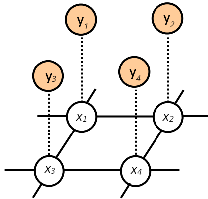
Abbildung 3-7: Markov Random Field mit Daten \mathbf{y}_i und Labels x_i (ähnlich Bishop, 2006)
