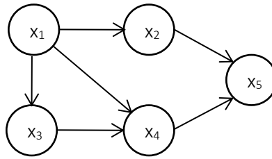
Abbildung 3-5: Gerichteter Graph für fünf Variablen
