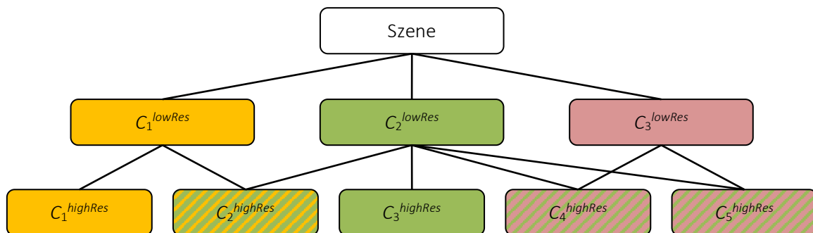
Abbildung 4-6: Semantisches Netz mit M:N Relationen.
