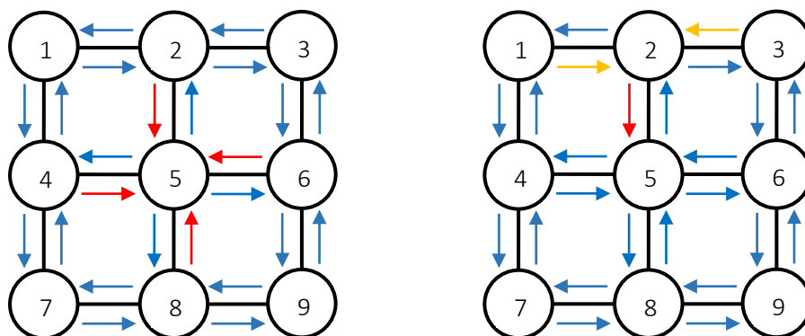
Abbildung 3-9: Nachrichtenübertragung (message passing) in einem ungerichteten Graphen mit regelmäßiger Gitterstruktur. Links: eingehende Nachrichten für Knoten 5 (rote Pfeile). Rechts: Abhängigkeit einer Nachricht (roter Pfeil) von anderen Nachrichten (orangene Pfeile).
