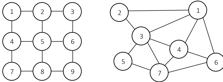
Abbildung 3-3: Nachbarschaftsgraphen; Links: Graph mit regelmäßiger Struktur; Rechts: Graph mit unregelmäßiger Struktur
