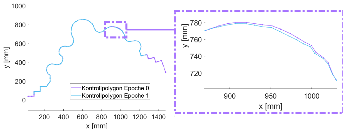
Abb. 7.49: Kontrollpolygone von Epoche 0 und Epoche 1 mit Deformation (2D-Fassadenstück).
