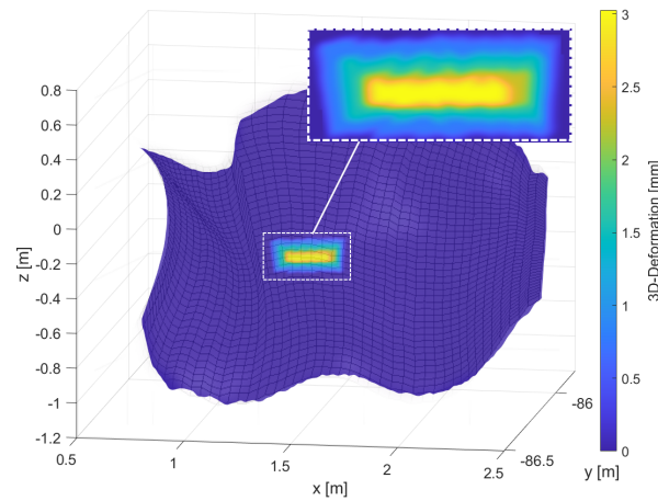
Abb. 7.56: 3D-Deformation korrespondierender B-Spline-Flächenpunkte von Epoche 0 und Epoche 1 ohne Messrauschen (Referenz-3D-Deformation, Gurkenblatt).
