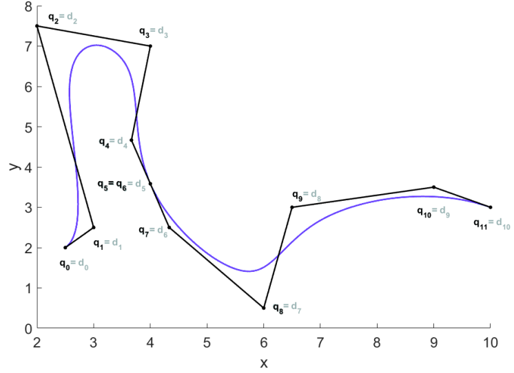
Abb. A.4: B-Spline-Kurve dritten Grades nach dritter Anwendung des Algorithmus von Böhm.
