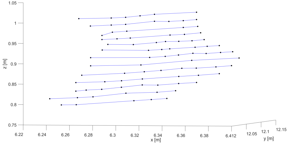
Abb. A.8: Kontrollpolygone.
