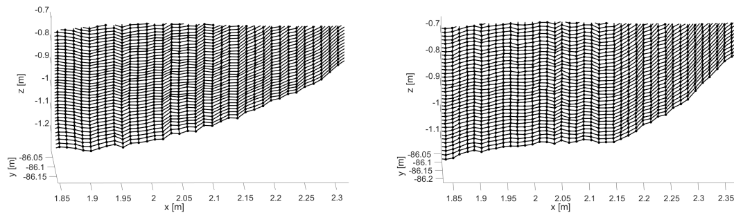
Abb. 7.14: Ausschnitt der Kontrollgitter von Gurkenblatt Epoche 0 (links) und Epoche 1 (rechts).
