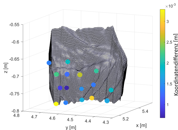
Abb. 7.33: Identische Punkte (Tontorso, Iteration 3).
