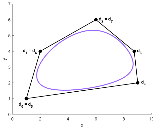
Abb. 2.15: Geschlossene periodische uniforme B-Spline-Kurven vom Grad 3.
