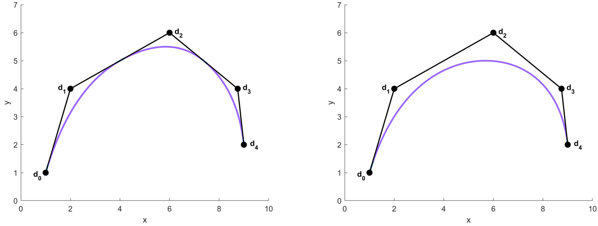
Abb. 2.16: Offene uniforme B-Spline-Kurven vom Grad 2 (links) und Grad 3 (rechts) (Aichinger und Schwieger 2022).
