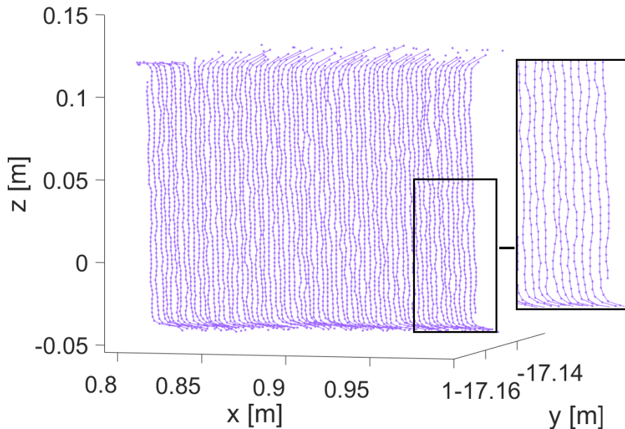
Abb. 4.6: Definierte Kontrollpolygone eines Laserscans einer Platte (Aichinger und Schwieger 2022).
